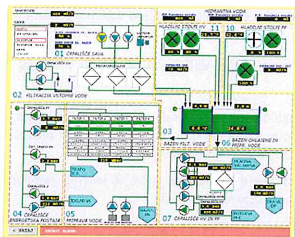
Slika 21: Primer nadzornega sistema ZPHV (Zaprti sistem hladilnih vod)
