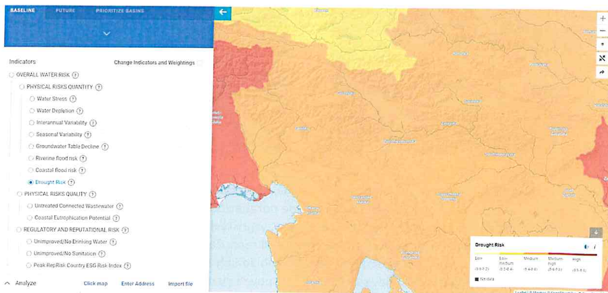
Slika 16: Tveganje za sušo, vir: Aqueduct Water Risk Atlas
