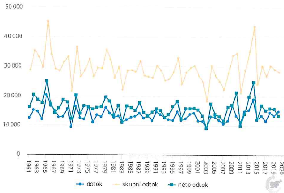
Slika 12: Letna rečna bilanca Slovenije (neto odtok kot razlika med skupnim odtokom in dotokom) Vir: ARSO, Kazalci okolja v Sloveniji. Povzeto po kazalcu MR02 – Višina morja, 2021
