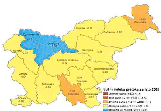
Slika 6: Sušni indeks pretoka za leto 2021 po regijah (vir ARSO)
