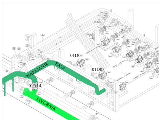
Slika 16: Avtomatiziran preklap Javornik - Sava
