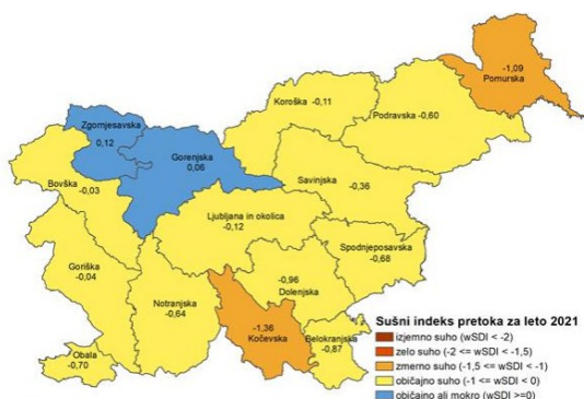
Slika 6: Sušni indeks pretoka za leto 2021 po regijah (vir ARSO)
