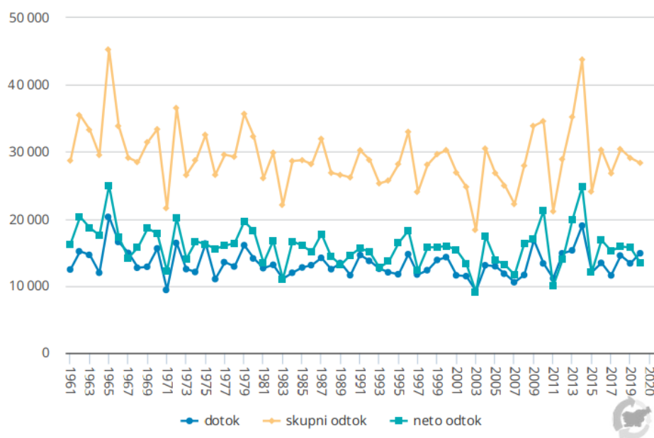
Slika 11: Letna rečna bilanca Slovenije (neto odtok kot razlika med skupnim odtokom in dotokom) Vir: ARSO, Kazalci okolja v Sloveniji. Povzeto po kazalcu MR02 – Višina morja, 2021
