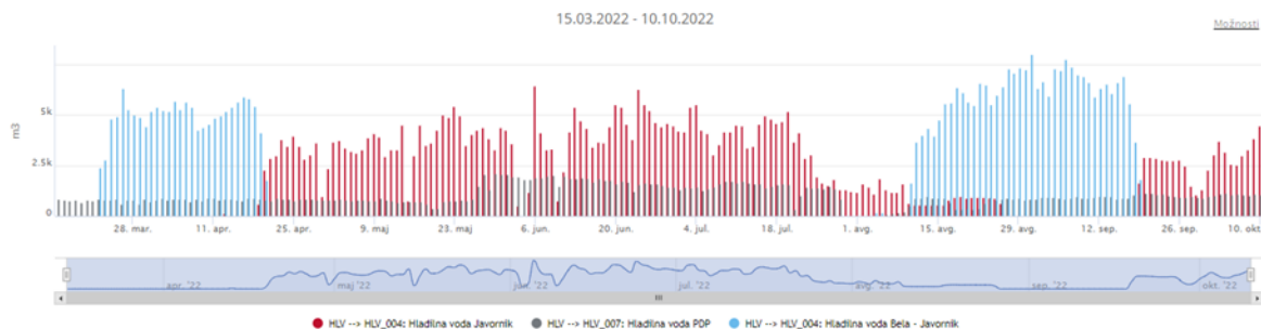
Slika 21: Merjenje porabe hladilne vode in prikaz preklopa na zajetje Sava
