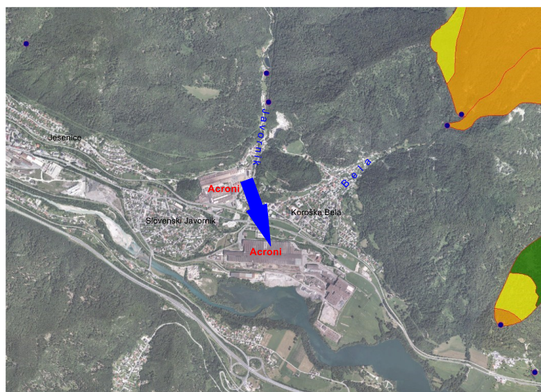
Slika 2: Vodovarstvena območja na obravnavanem območju in smer toka podzemne vode z območja naprave Acroni (vir: Atlas Okolja; DOF in VVO)
