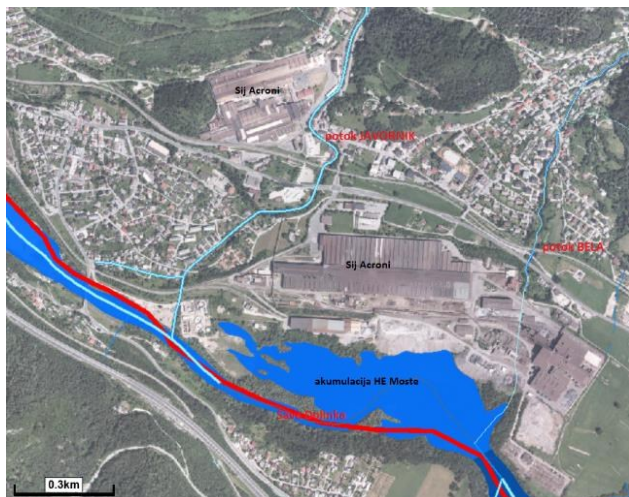
Slika 1: Površinske vode na območju Sij Acroni. (vir: Atlas okolja, oktober 2016)
