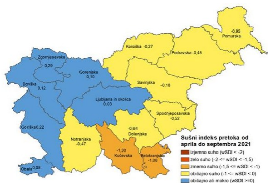
Slika 7: Polletni sušni indeks pretoka od aprila do septembra 2021 po regijah (vir ARSO)
